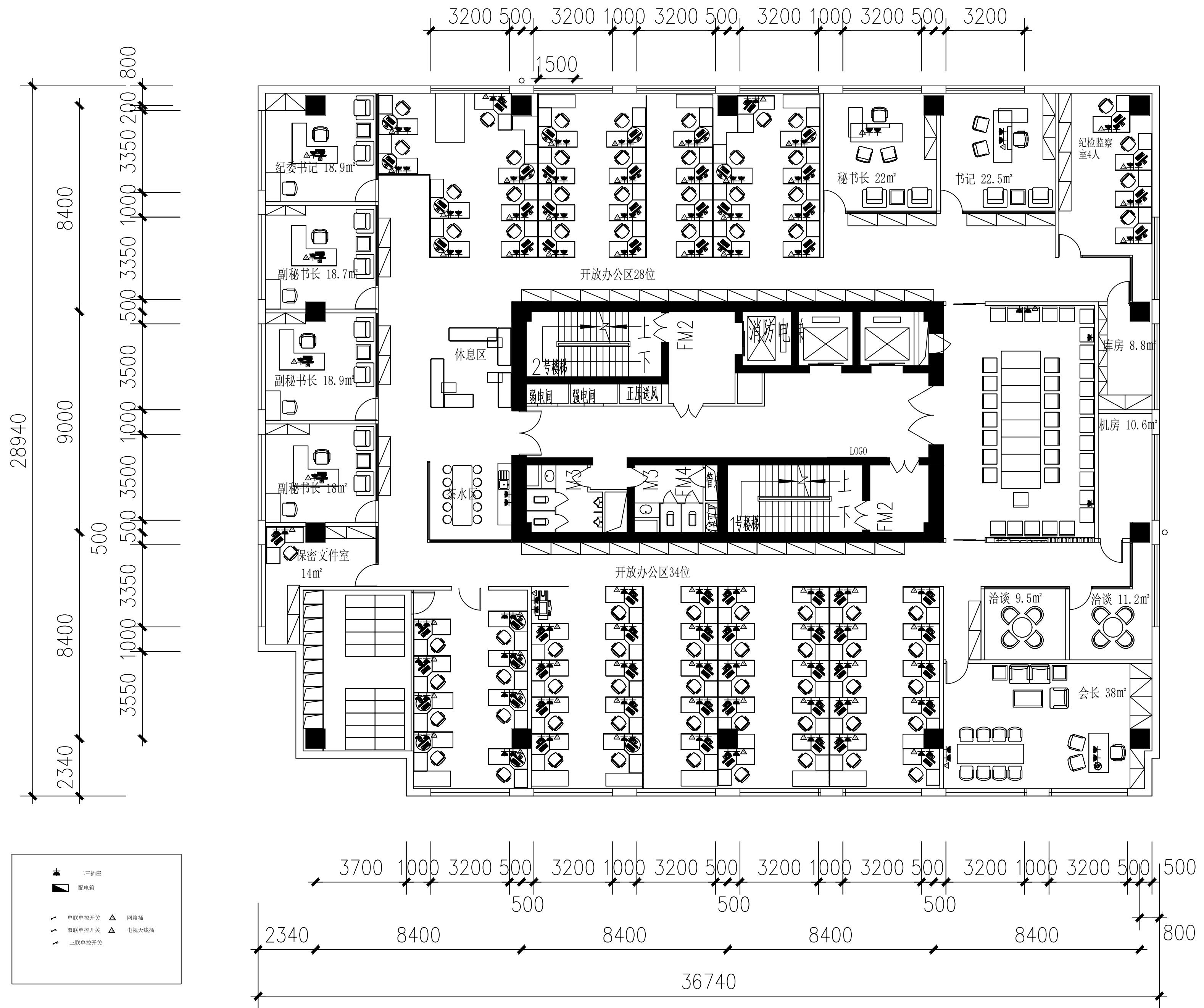
A座8层插座网络点位图
